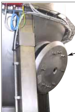
VALVOLA RELIEF PER POLVERI ST1-ST2 VANNE RELIEF POUR POUSSIÈRES ST1-ST2 RELIEF VALVE FOR DUSTS ST1-ST2 RELIEF- VENTIL FÜR ST1- ST2- STÄUBE VALVULA RELIEF PARA POLVOS ST1-ST2
